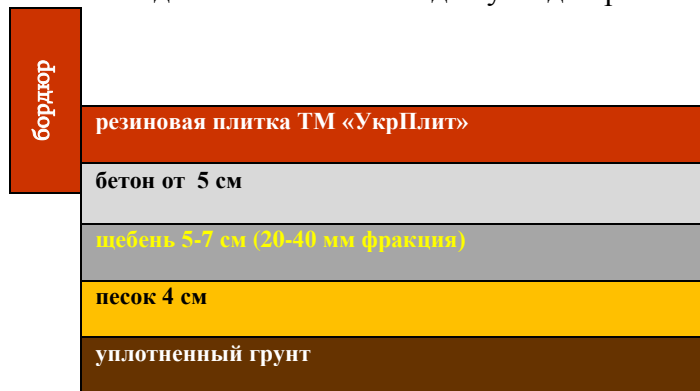
Рис.1 – Подготовка основания для укладки резиновой плитки на бетон:
